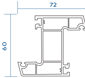
Z Mullion VGC-601-T03
