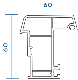
Fly Mullion VGC-601-T02
