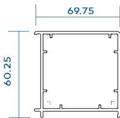
Square Corner VGA-160-A04
