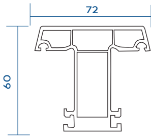
Casement T Mullion VGC-601-T01
