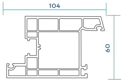
Inward Door Sash VGC-601-S03
