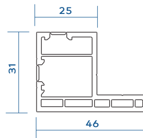
Grill Frame VGA-160-A01
